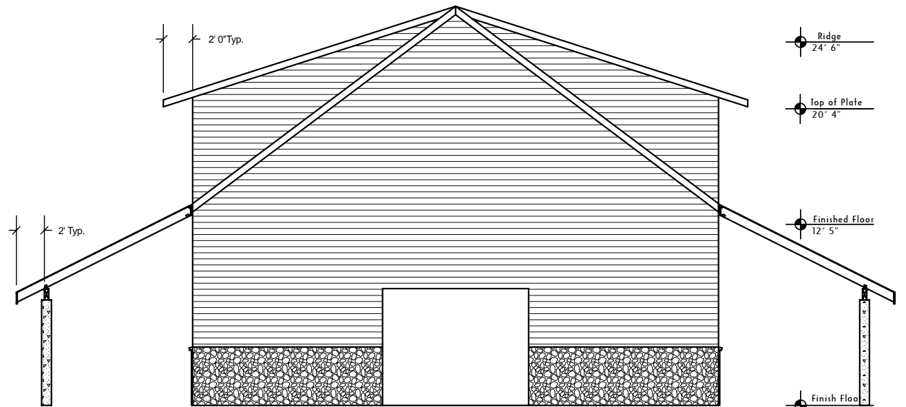
B 3 ELEVATION
