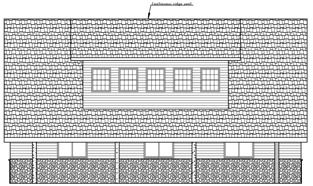
A 3 ELEVATION
