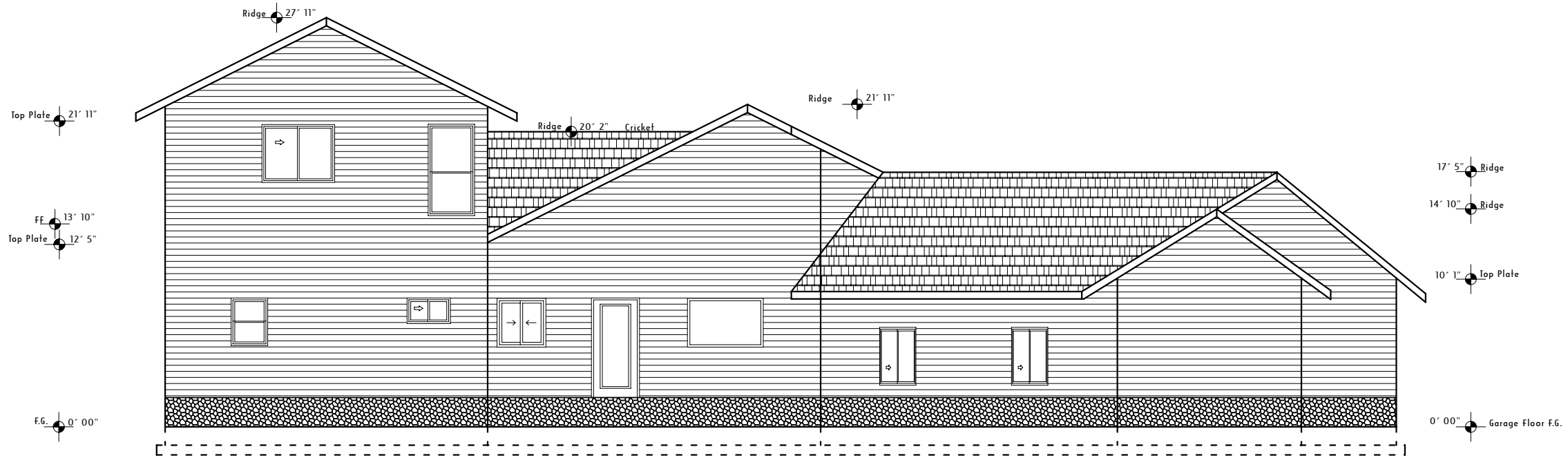
B 4 ELEVATION
